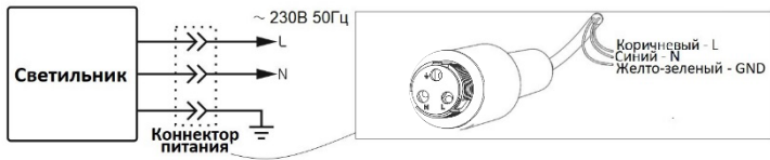
Рисунок 2 Схема подключения светильника
